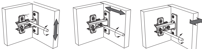
Регулирование зазоров и положения дверей с петлями по высоте, ширине, глубине
