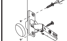
Регулирование зазоров и положения дверей с петлями по высоте, ширине, глубине
