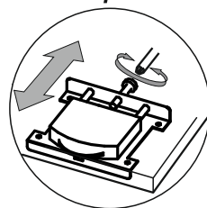
Регулировка створки
