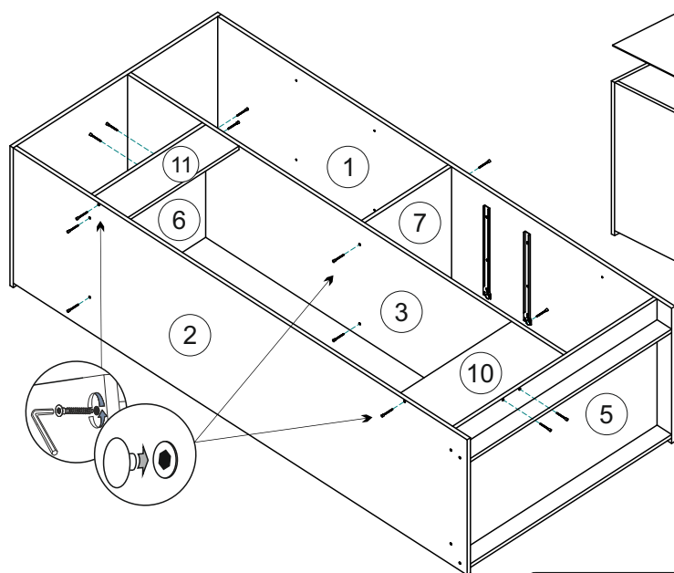
схема крепления евровинта
