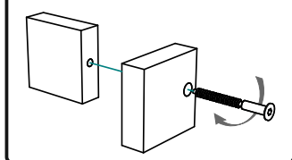
схема крепления евровинта
