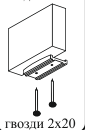
схема монтажа подпятника
