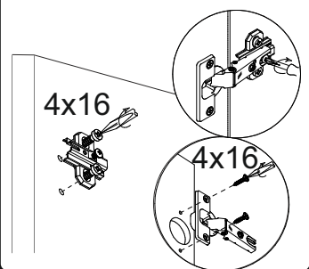
схема монтажа петель
