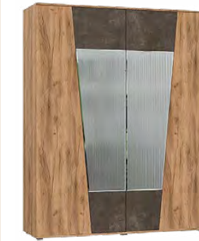
Шкаф 4-х створчатый (ШхВхГ) 1800х2236х546 мм
