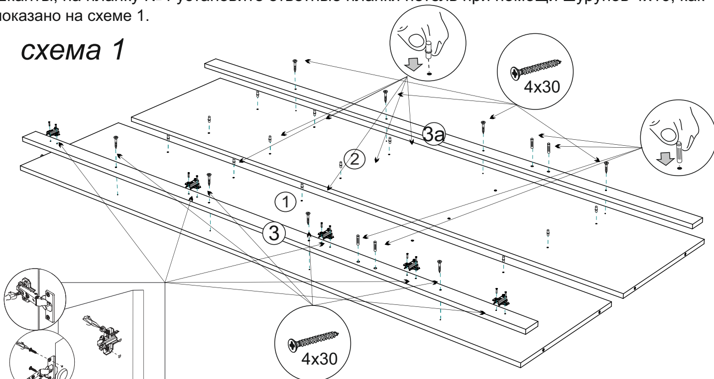
Крепление ответной планки петли
