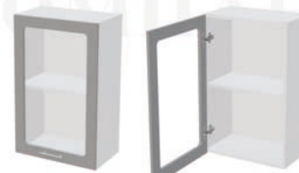
Корпус: ШБ500 / ШВС500 500x718x283 (ШxBxГ) Фасад: ШВС500 497x715x16 (ШxBxГ) - 1 шт.
