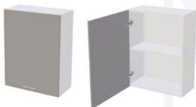
Корпус: ШБ1Д600 / ШВС1Д600 600x718x283 (ШxBxГ) Фасад: ШН1Д600 / ШНМ1Д600 / ШВ1Д600 597x715x16 (ШxBxГ) - 1 шт.
