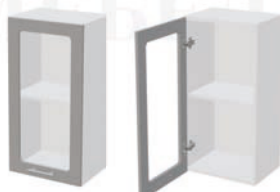
Корпус: ШБ400 / ШВС400 400x718x283 (ШxBxГ) Фасад: ШВС400 397x715x16 (ШxBxГ) - 1 шт.
