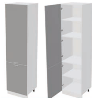
Корпус: ШП600-2 600x2140x553 (ШxBxГ) Фасад: ШП600-2 597x1317x16 (ШxBxГ) - 1 шт. 597x715x16 (ШxBxГ) - 1 шт.
