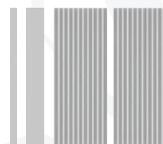
ШБУП600 34x715x16 - 1 шт. 90x715x16 - 1 шт. 262x715x16 - 2 шт.
