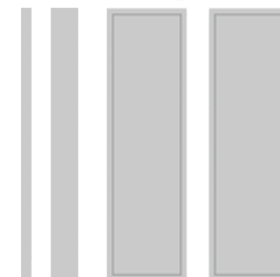
ШВУП600x900 34x895x16 - 1 шт. 90x895x16 - 1 шт. 262x895x16 - 2 шт.
