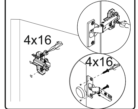
схема монтажа петли
