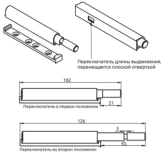
Схема установки и регулировки толкателя!
