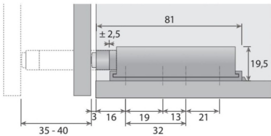
Схема монтажа, демонтажа направляющих
