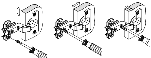
Регулирование зазоров и положения дверей с петлями
