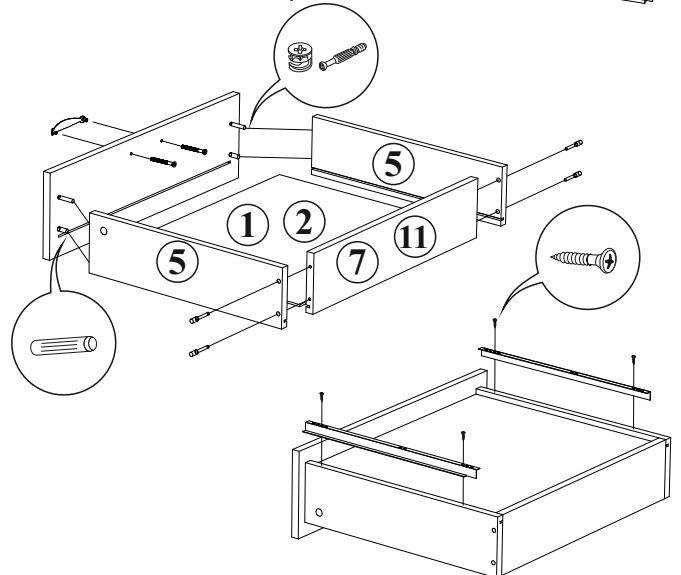
Сборка ящика
