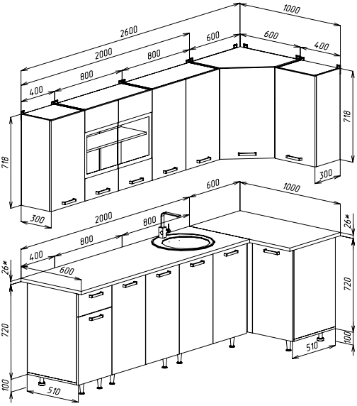
РИО NEW 2,6x1,0 (490)
