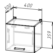
Корпус: ШВГ400/360 (ШхВхГ) 400х359х300 мм Фасад: ЛДСП ФАСАД РИО NEW ШВГ400/360 / ШВГА 400/360
