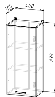
Корпус: ШВ400/900 / ШВС400/900 (ШхВхГ) 400х898х300 мм Фасад: ЛДСП ФАСАД РИО NEW ШВ400/900
