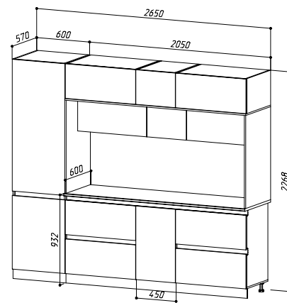
ЦЕНТРАЛЬНАЯ СЕКЦИЯ 2050 (С МЕСТОМ ПОД МП)+ПЕНАЛ (ШхВхГ) 2650х2268х600 мм
