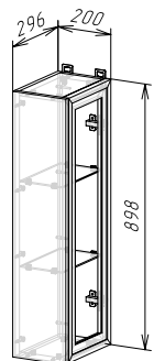
Корпус: ШВТД200/900 (ШхВхГ) 200x898x300 мм Фасад: ЛДСП ФАСАД РИО NEW ШВТД200/900
