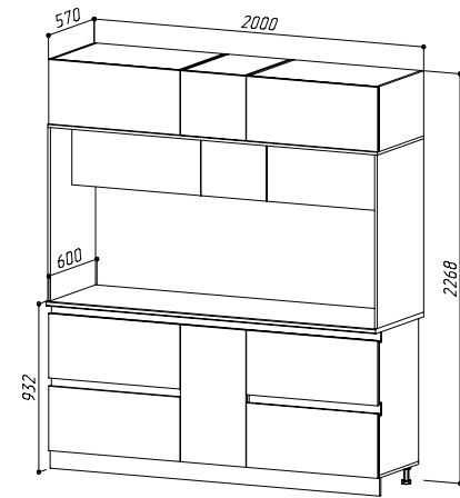
ЦЕНТРАЛЬНАЯ СЕКЦИЯ 2000 2000×2268×600 мм
