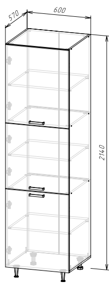
Корпус: ШП600/ШП600-1/ШП600-2 (ШхВхГ) 600x2140x570 мм Фасад: ЛДСП ФАСАД РИО NEW ШП600-1
