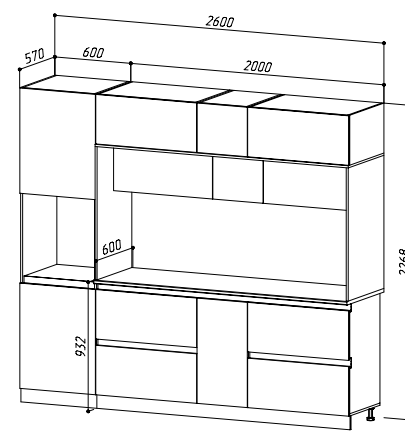
ЦЕНТРАЛЬНАЯ СЕКЦИЯ 2000+ПЕНАЛ ДЛЯ ВСТРАИВАЕМОЙ БЫТОВОЙ ТЕХНИКИ (ШхВхГ) 2600х2268х600 мм
