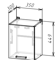
Корпус: ШВГ350/450 (ШхВхГ) 350х449х300 мм Фасад: ЛДСП ФАСАД РИО NEW ШВГ350/450
