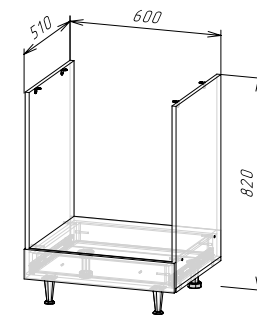
Корпус: ШНВТ600(490) (ШхВхГ) 600x820x510 мм Фасад: ЛДСП ФАСАД РИО NEW ШНВТ600
