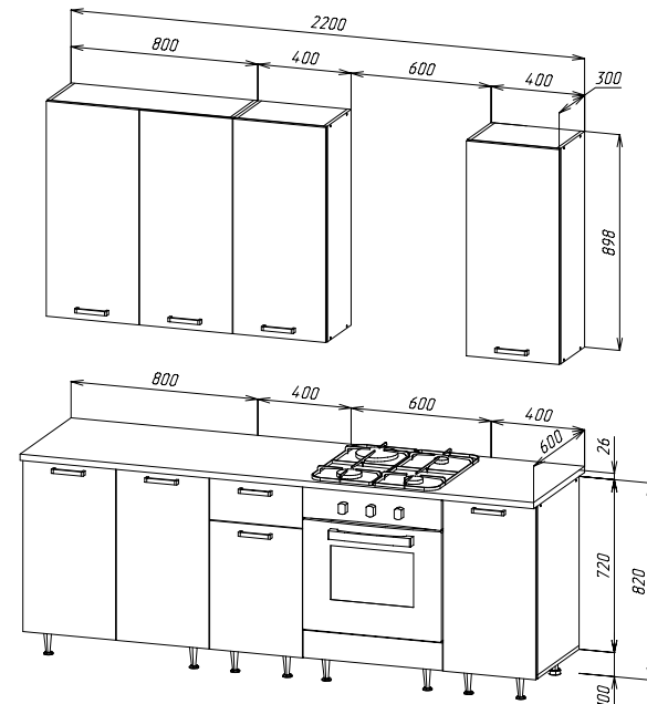
РИО NEW 2,2/900 (490) КОМПОНОВКА #2
