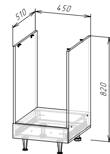
Корпус: ШНВТ450(490) (ШхВхГ) 450x820x510 мм Фасад: ЛДСП ФАСАД РИО NEW ШНВТ450
