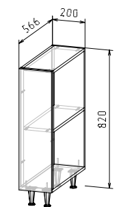
Корпус: ТР 820 (ШхВхГ) 200x820x566 мм
