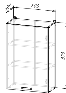
Корпус: ШВ600/900 / ШВС600/900 / ШВ1Д600/900 / ШВС1Д600/900 (ШхВхГ) 600х898х300 мм Фасад: ЛДСП ФАСАД РИО NEW ШВ1Д600/900
