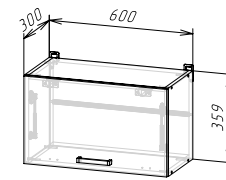
Корпус: ШВГ600/360 / ШВГС600/360 (ШхВхГ) 600х359х300 мм Фасад: ЛДСП ФАСАД РИО NEW ШВГ600/360 / ШВГА 600/360
