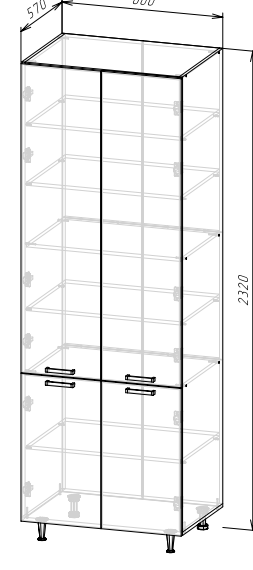
Корпус: ШПВ800/ШПВС800 (ШхВхГ) 800x2320x570 мм Фасад: ЛДСП ФАСАД РИО NEW ШПВ800
