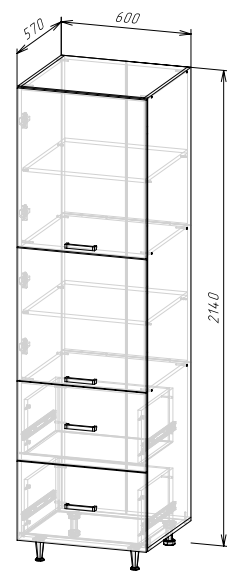
Корпус: ШП2Я600/ШП2Я600-1/ ШП2Я600-2 (ШхВхГ) 600x2140x570 мм Фасад: ЛДСП ФАСАД РИО NEW ШП2Я600-1
