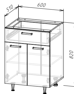
Корпус: ШН1Я600/ШН1Д1Я600(490) (ШхВхГ) 600x820x510 мм Фасад: ЛДСП ФАСАД РИО NEW ШН1Я600
