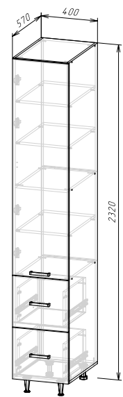
Корпус: ШПВ2Я400/ШПВ2Я400-1 (ШхВхГ) 400x2320x570 мм Фасад: ЛДСП ФАСАД РИО NEW ШПВ2Я400-1
