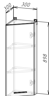
Корпус: ШВТД300/900 (ШхВхГ) 300x898x300 мм Фасад: ЛДСП ФАСАД РИО NEW ШВТД300/900
