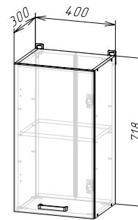
Корпус: ШВ400/ШВС400 (ШхВхГ) 400x718x300 мм Фасад: ЛДСП ФАСАД РИО NEW ШВ400/ШН400
