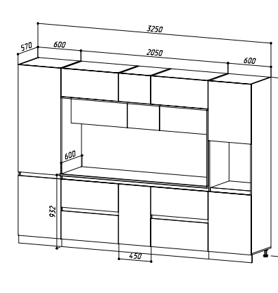
ЦЕНТРАЛЬНАЯ СЕКЦИЯ 2050 (С МЕСТОМ ПОД МП)+ПЕНАЛ+ПЕНАЛ ДЛЯ ВСТРАИВАЕМОЙ БЫТОВОЙ ТЕХНИКИ (ШхВхГ) 3250х2268х600 мм
