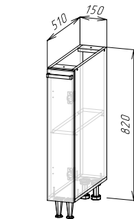
Корпус: ШН150(490) (ШхВхГ) 150х820х510 мм Фасад: ЛДСП ФАСАД РИО NEW ШВ150/ШН150
