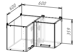
Корпус: ШВУП600/360 (ШхВхГ) 600x359x600 мм Фасад: ЛДСП ФАСАД РИО NEW ШВУП600/360
