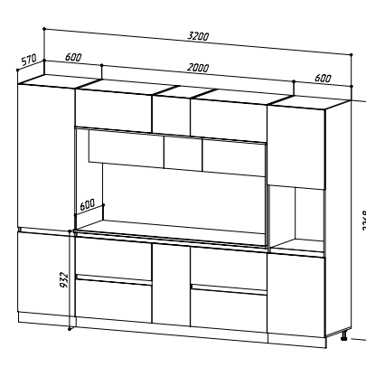
ЦЕНТРАЛЬНАЯ СЕКЦИЯ 2000+ПЕНАЛ+ПЕНАЛ ДЛЯ ВСТРАИВАЕМОЙ БЫТОВОЙ ТЕХНИКИ (ШхВхГ) 3200х2268х600 мм
