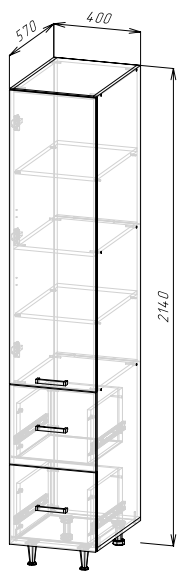
Корпус: ШП2Я400/ШП2Я400-1 (ШхВхГ) 400x2140x570 мм Фасад: ЛДСП ФАСАД РИО NEW ШП2Я400-1
