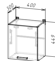
Корпус: ШВГ400/450 (ШхВхГ) 400х449х300 мм Фасад: ЛДСП ФАСАД РИО NEW ШВГ400/450
