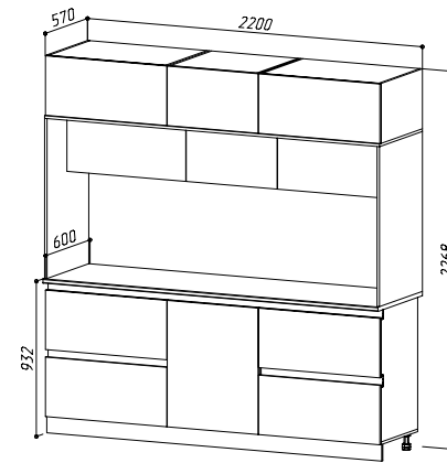
ЦЕНТРАЛЬНАЯ СЕКЦИЯ 2200 (ШхВхГ) 2200х2268х600 мм
