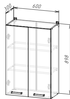
Корпус: ШВ600/900 / ШВС600/900 / ШВ1Д600/900 / ШВС1Д600/900 (ШхВхГ) 600х898х300 мм Фасад: ЛДСП ФАСАД РИО NEW ШВ600/900
