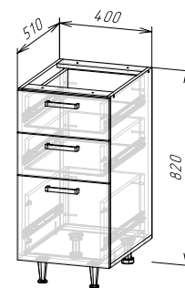
Корпус: ШНЗЯ400(490) (ШхВхГ) 400x820x510 мм Фасад: ЛДСП ФАСАД РИО NEW ШНЗЯ400
