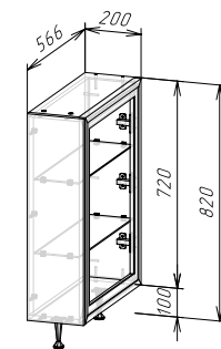
Корпус: ШНТД200 (ШхВхГ) 200x820x566 мм Фасад: ЛДСП ФАСАД РИО NEW ШВТД200/ШНТД200
