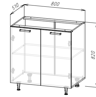
Корпус: ШН800(490) (ШхВхГ) 800х820х510 мм Фасад: ЛДСП ФАСАД РИО NEW ШВ800/ШН800/ШНМ800
