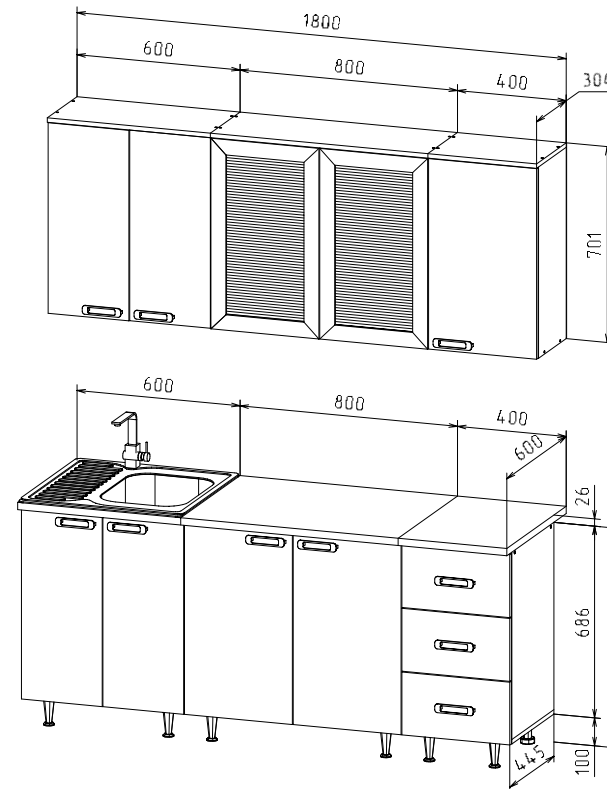
ЛДСП КУХНЯ "КАТЯ" 1,8м
