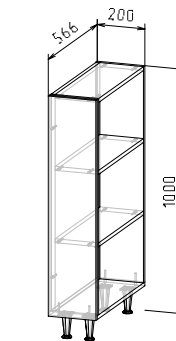
Корпус: ТР 1000 (ШхВхГ) 200x1000x566 мм
