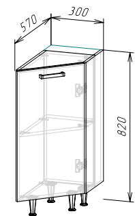
Корпус: ШНТД300 (ШхВхГ) 300x820x570 мм Фасад: ЛДСП ФАСАД РИО NEW ШНТД300
