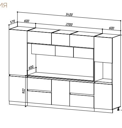
ЦЕНТРАЛЬНАЯ СЕКЦИЯ 2200+ПЕНАЛ+ПЕНАЛ ДЛЯ ВСТРАИВАЕМОЙ БЫТОВОЙ ТЕХНИКИ (ШхВхГ) 3400х2268х600 мм
