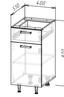
Корпус: ШН1Я400(490) (ШхВхГ) 400х820х510 мм Фасад: ЛДСП ФАСАД РИО NEW ШН1Я400
