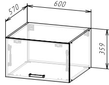
Корпус: ШВГА600/360 (ШхВхГ) 600x359x570 мм Фасад: ЛДСП ФАСАД РИО NEW ШВГ600/360 / ШВГА 600/360
