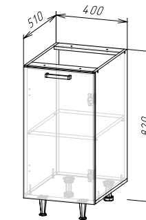
Корпус: ШН400(490) (ШхВхГ) 400х820х510 мм Фасад: ЛДСП ФАСАД РИО NEW ШВ400/ШН400
