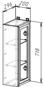
Корпус: ШВТД200 (ШхВхГ) 200x718x300 мм Фасад: ЛДСП ФАСАД РИО NEW ШВТД200/ШНТД200
