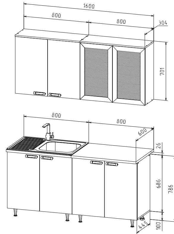
ЛДСП КУХНЯ "КАТЯ" 1,6м
