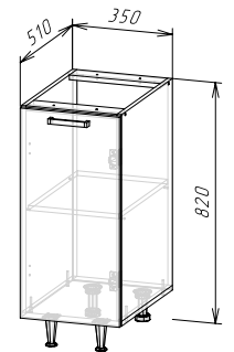
Корпус: ШН350(490) (ШхВхГ) 350х820х510 мм Фасад: ЛДСП ФАСАД РИО NEW ШВ350/ШН350
