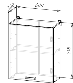
Корпус: ШВ600/ШВС600/ ШВ1Д600/ШВС1Д600 (ШхВхГ) 600x718x300 мм Фасад: ЛДСП ФАСАД РИО NEW ШВ1Д600/ШН1Д600/ШНМ1Д600
