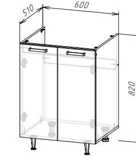
Корпус: ШНМ600/ШНМ1Д600 (490) (ШхВхГ) 600х820х510 мм Фасад: ЛДСП ФАСАД РИО NEW ШВ600/ШН600/ШНМ600
