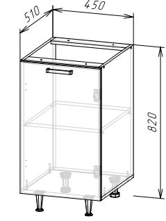
Корпус: ШН450(490) (ШхВхГ) 450х820х510 мм Фасад: ЛДСП ФАСАД РИО NEW ШВ450/ШН450
