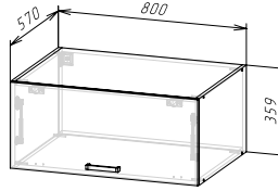
Корпус: ШВГА800/360 (ШхВхГ) 800x359x570 мм Фасад: ЛДСП ФАСАД РИО NEW ШВГ800/360 / ШВГА 800/360
