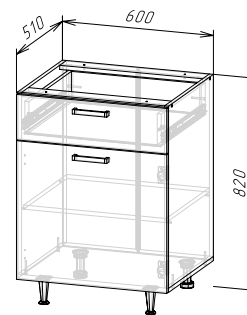
Корпус: ШН1Я600/ШН1Д1Я600(490) (ШхВхГ) 600x820x510 мм Фасад: ЛДСП ФАСАД РИО NEW ШН1Д1Я600
