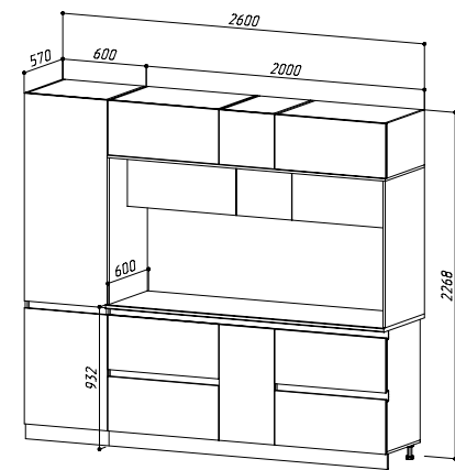
ЦЕНТРАЛЬНАЯ СЕКЦИЯ 2000+ПЕНАЛ (ШхВхГ) 2600х2268х600 мм
