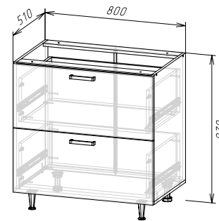
Корпус: ШН2ЯГ800(490) (ШхВхГ) 800x820x510 мм Фасад: ЛДСП ФАСАД РИО NEW ШН2ЯГ800
