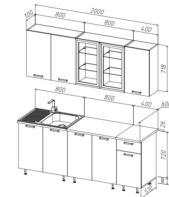
КУХНЯ РИО NEW 2,0 (490) КОМПОНОВКА #1
