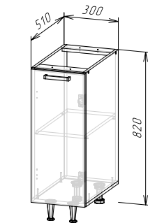
Корпус: ШН300(490) (ШхВхГ) 300х820х510 мм Фасад: ЛДСП ФАСАД РИО NEW ШВ300/ШН300
