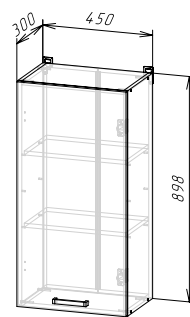
Корпус: ШВ450/ШВС450 (ШхВхГ) 450х898х300 мм Фасад: ЛДСП ФАСАД РИО NEW ШВ450/900
