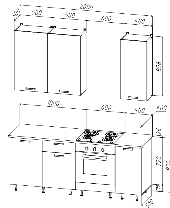
РИО NEW 2,0/900 (490) КОМПОНОВКА #2
