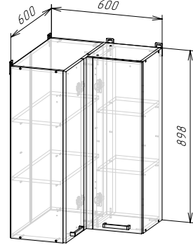
Корпус: ШВУП600/900 (ШхВхГ) 600x898x600 мм Фасад: ЛДСП ФАСАД РИО NEW ШВУП600/900
