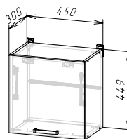
Корпус: ШВГ450/450 (ШхВхГ) 450х449х300 мм Фасад: ЛДСП ФАСАД РИО NEW ШВГ450/450
