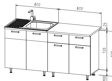
ЛДСП КУХНЯ ГРАНД 1,6 (490)
