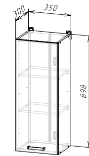
Корпус: ШВ350/900 (ШхВхГ) 350х898х300 мм Фасад: ЛДСП ФАСАД РИО NEW ШВ350/900
