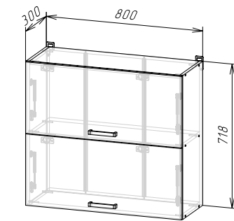
Корпус: ШВГ800/ШВГС800 (ШхВхГ) 800х718х300 мм Фасад: ЛДСП ФАСАД РИО NEW ШВГ800
