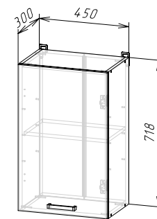
Корпус: ШВ450/ШВС450 (ШхВхГ) 450x718x300 мм Фасад: ЛДСП ФАСАД РИО NEW ШВ450/ШН450
