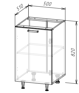
Корпус: ШН500(490) (ШхВхГ) 500х820х510 мм Фасад: ЛДСП ФАСАД РИО NEW ШВ500/ШН500/ШНМ500
