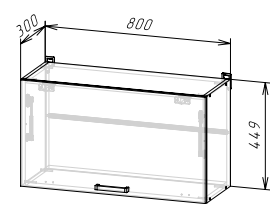
Корпус: ШВГ800/450 (ШхВхГ) 800х449х300 мм Фасад: ЛДСП ФАСАД РИО NEW ШВГ800/450
