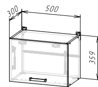
Корпус: ШВГ500/360 / ШВГС500/360 (ШхВхГ) 500х359х300 мм Фасад: ЛДСП ФАСАД РИО NEW ШВГ500/360 / ШВГА 500/360
