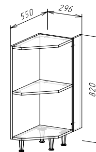
Корпус: ШНТ300 (ШхВхГ) 296x820x550 мм
