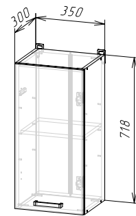
Корпус: ШВ350 (ШхВхГ) 350x718x300 мм Фасад: ЛДСП ФАСАД РИО NEW ШВ350/ШН350
