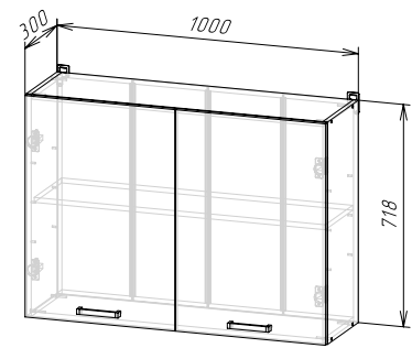
Корпус: ШВ1000/ШВС1000 (ШхВхГ) 1000х718х300 мм Фасад: ЛДСП ФАСАД РИО NEW ШВ1000
