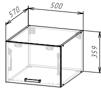
Корпус: ШВГА500/360 (ШхВхГ) 500x359x570 мм Фасад: ЛДСП ФАСАД РИО NEW ШВГ500/360 / ШВГА 500/360
