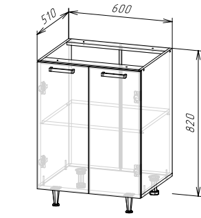
Корпус: ШН600/ШН1Д600 (490) (ШхВхГ) 600х820х510 мм Фасад: ЛДСП ФАСАД РИО NEW ШВ600/ШН600/ШНМ600
