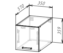
Корпус: ШВГА350/360 (ШхВхГ) 350x359x570 мм Фасад: ЛДСП ФАСАД РИО NEW ШВГ350/360 / ШВГА 350/360
