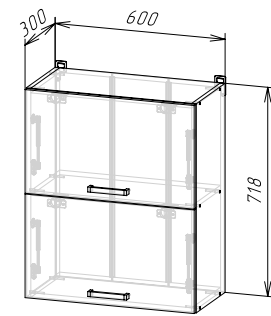
Корпус: ШВГ600/ШВГС600 (ШхВхГ) 600х718х300 мм Фасад: ЛДСП ФАСАД РИО NEW ШВГ600
