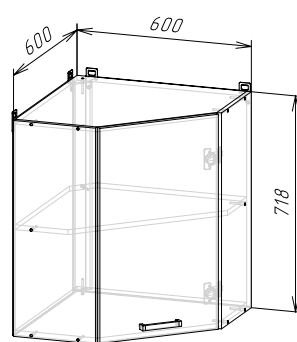
Корпус: ШВУ600 / ШВУС600 (ШхВхГ) 600x718x600 мм Фасад: ЛДСП ФАСАД РИО NEW ШВУ600
