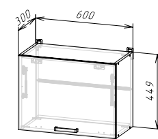
Корпус: ШВГ600/450 (ШхВхГ) 600х449х300 мм Фасад: ЛДСП ФАСАД РИО NEW ШВГ600/450
