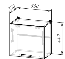
Корпус: ШВГ500/450 (ШхВхГ) 500х449х300 мм Фасад: ЛДСП ФАСАД РИО NEW ШВГ500/450
