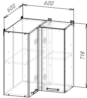
Корпус: ШВУП600 (ШхВхГ) 600x718x600 мм Фасад: ЛДСП ФАСАД РИО NEW ШВУП600
