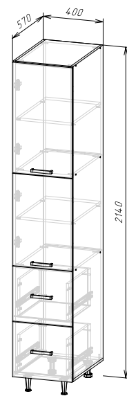
Корпус: ШП2Я400/ШП2Я400-1 (ШхВхГ) 400x2140x570 мм Фасад: ЛДСП ФАСАД РИО NEW ШП2Я400
