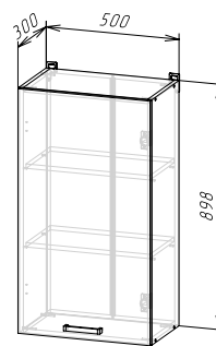
Корпус: ШВ500/900 / ШВС500/900 (ШхВхГ) 500х898х300 мм Фасад: ЛДСП ФАСАД РИО NEW ШВ500/900
