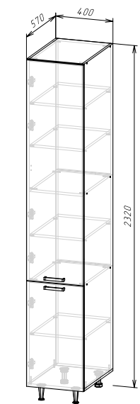
Корпус: ШПВ400/ШПВ400-1 (ШхВхГ) 400x2320x570 мм Фасад: ЛДСП ФАСАД РИО NEW ШПВ400-1
