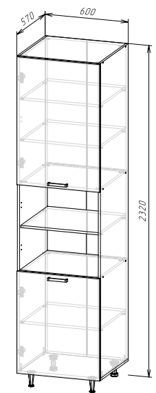
Корпус: ШПВ600/ШПВ600-1/ШПВ600-2 (ШхВхГ) 600x2320x570 мм Фасад: ЛДСП ФАСАД РИО NEW ШПВ600
