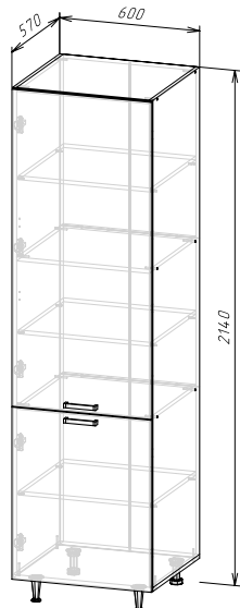
Корпус: ШП600/ШП600-1/ШП600-2 (ШхВхГ) 600x2140x570 мм Фасад: ЛДСП ФАСАД РИО NEW ШП600-2
