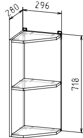
Корпус: ШВТ 300 (ШхВхГ) 296x718x280 мм
