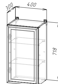
Корпус: ШВ400/ШВС400 (ШхВхГ) 400х718х300 мм Фасад: ФАСАД (РАМКА AGT ШВС400)
