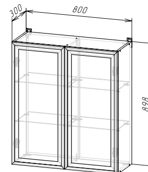
Корпус: ШВСП 800/900 НИКОЛЬ (ШхВхГ) 800х898х300 мм Фасад: ФАСАД (РАМКА AGT ШВС800/900)
