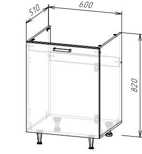
Корпус: ШНМ600/ШНМ1Д600 (490) (ШхВхГ) 600х820х510 мм Фасад: ЛДСП ФАСАД РИО NEW ШВ1Д600/ШН1Д600/ШНМ1Д600
