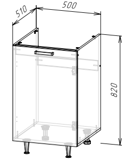
Корпус: ШНМ500(490) (ШхВхГ) 500х820х510 мм Фасад: ЛДСП ФАСАД РИО NEW ШВ500/ШН500/ШНМ500
