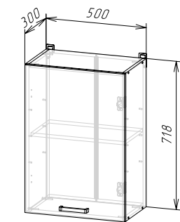
Корпус: ШВ500/ШВС500 (ШхВхГ) 500x718x300 мм Фасад: ЛДСП ФАСАД РИО NEW ШВ500/ШН500/ШНМ500
