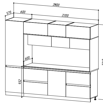
ЦЕНТРАЛЬНАЯ СЕКЦИЯ 2200+ПЕНАЛ (ШхВхГ) 2800х2268х600 мм
