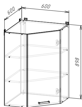
Корпус: ШВУ600/900 / ШВУС600/900 (ШхВхГ) 600x898x600 мм Фасад: ЛДСП ФАСАД РИО NEW ШВУ600/900
