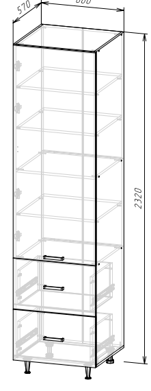
Корпус: ШПВ2Я600/ШПВ2Я600-1/ ШПВ2Я600-2 (ШхВхГ) 600x2320x570 мм Фасад: ЛДСП ФАСАД РИО NEW ШПВ2Я600-2
