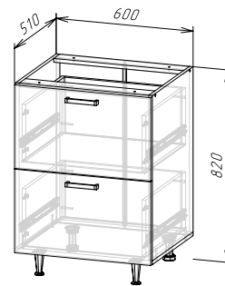
Корпус: ШН2ЯГ600(490) (ШхВхГ) 600x820x510 мм Фасад: ЛДСП ФАСАД РИО NEW ШН2ЯГ600
