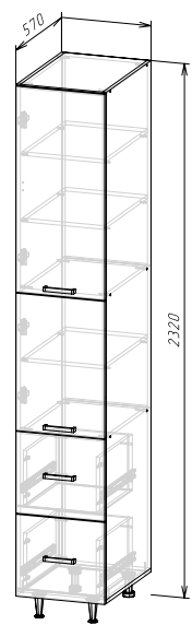
Корпус: ШПВ2Я400/ШПВ2Я400-1 (ШхВхГ) 400x2320x570 мм Фасад: ЛДСП ФАСАД РИО NEW ШПВ2Я400
