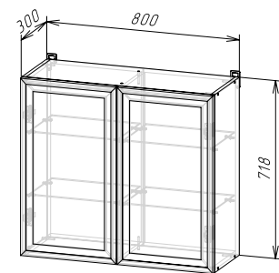
Корпус: ШВСП 800 НИКОЛЬ (ШхВхГ) 800х718х300 мм Фасад: ФАСАД (РАМКА AGT ШВС800)
