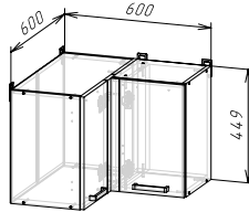
Корпус: ШВУП600/450 (ШхВхГ) 600x449x600 мм Фасад: ЛДСП ФАСАД РИО NEW ШВУП600/450
