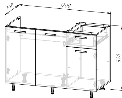
Корпус: ШН1Я1200(490) (ШхВхГ) 1200x820x510 мм Фасад: ЛДСП ФАСАД РИО NEW ШН1Я1200
