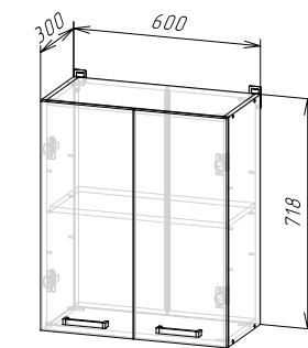
Корпус: ШВ600/ШВС600/ ШВ1Д600/ШВС1Д600 (ШхВхГ) 600x718x300 мм Фасад: ЛДСП ФАСАД РИО NEW ШВ600/ШН600/ШНМ600
