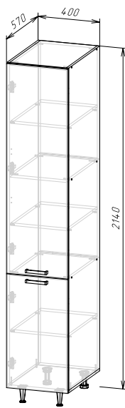
Корпус: ШП400/ШП400-1 (ШхВхГ) 400x2140x570 мм Фасад: ЛДСП ФАСАД РИО NEW ШП400-1
