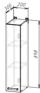
Корпус: ШВ200/900 (ШхВхГ) 200х898х300 мм Фасад: ЛДСП ФАСАД РИО NEW ШВ200/900
