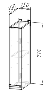
Корпус: ШВ150 (ШхВхГ) 150x718x300 мм Фасад: ЛДСП ФАСАД РИО NEW ШВ150/ШН150
