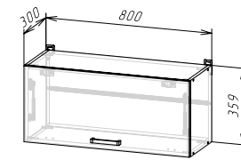
Корпус: ШВГ800/360 / ШВГС800/360 (ШхВхГ) 800х359х300 мм Фасад: ЛДСП ФАСАД РИО NEW ШВГ800/360 / ШВГА 800/360
