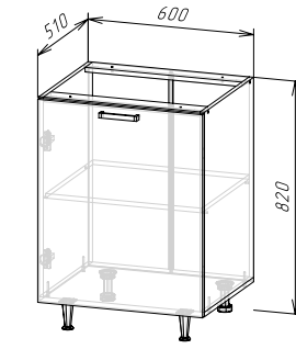
Корпус: ШН600/ШН1Д600 (490) (ШхВхГ) 600х820х510 мм Фасад: ЛДСП ФАСАД РИО NEW ШВ1Д600/ШН1Д600/ШНМ1Д600
