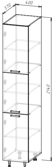
Корпус: ШП400/ШП400-1 (ШхВхГ) 400x2140x570 мм Фасад: ЛДСП ФАСАД РИО NEW ШП400
