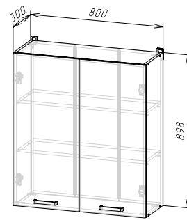
Корпус: ШВ800/900/ШВС800/900 (ШхВхГ) 800х898х300 мм Фасад: ЛДСП ФАСАД РИО NEW ШВ800/900
