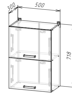
Корпус: ШВГ500/ШВГС500 (ШхВхГ) 500х718х300 мм Фасад: ЛДСП ФАСАД РИО NEW ШВГ500
