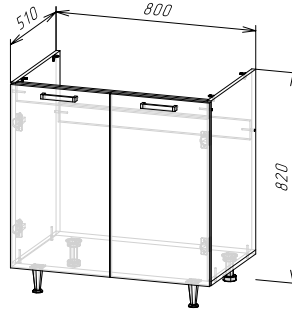
Корпус: ШНМ800(490) (ШхВхГ) 600х820х510 мм Фасад: ЛДСП ФАСАД РИО NEW ШВ800/ШН800/ШНМ800
