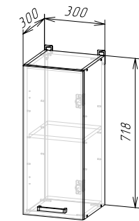
Корпус: ШВ300/ШВС300 (ШхВхГ) 300x718x300 мм Фасад: ЛДСП ФАСАД РИО NEW ШВ300/ШН300
