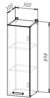
Корпус: ШВ300/900 / ШВС300/900 (ШхВхГ) 300х898х300 мм Фасад: ЛДСП ФАСАД РИО NEW ШВ300/900
