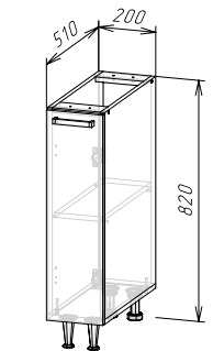
Корпус: ШН200(490) (ШхВхГ) 200х820х510 мм Фасад: ЛДСП ФАСАД РИО NEW ШВ200/ШН200
