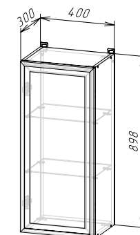
Корпус: ШВ400/900 / ШВС400/900 (ШхВхГ) 400х898х300 мм Фасад: ФАСАД (РАМКА AGT ШВС400/900)
