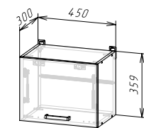
Корпус: ШВГ450/360 (ШхВхГ) 450х359х300 мм Фасад: ЛДСП ФАСАД РИО NEW ШВГ450/360 / ШВГА 450/360
