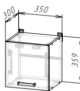
Корпус: ШВГ350/360 (ШхВхГ) 350х359х300 мм Фасад: ЛДСП ФАСАД РИО NEW ШВГ350/360 / ШВГА 350/360
